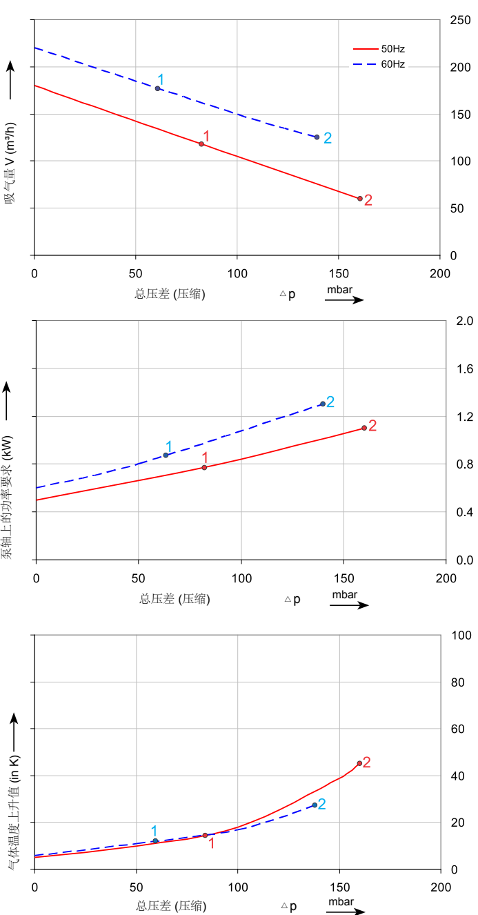
压力性能曲线
