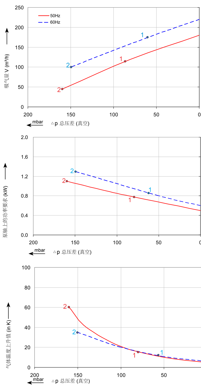
真空性能曲线
