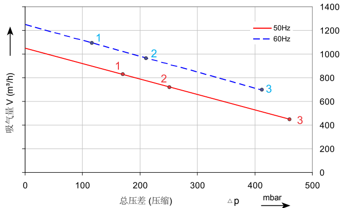
压力性能曲线
