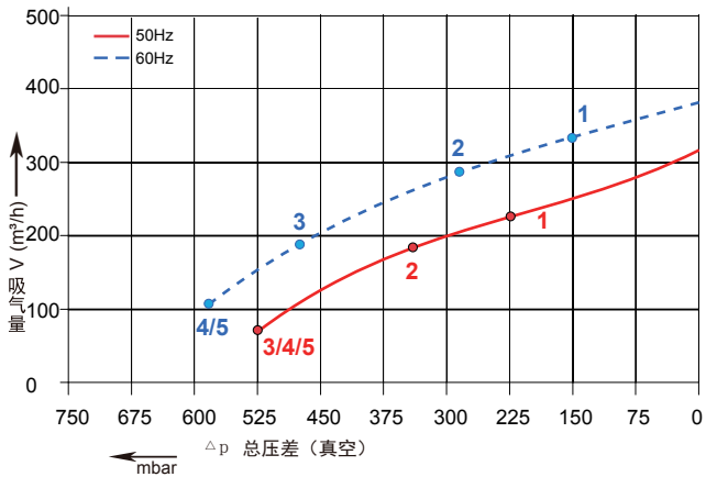
真空性能曲线
