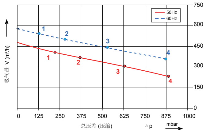
压力性能曲线
